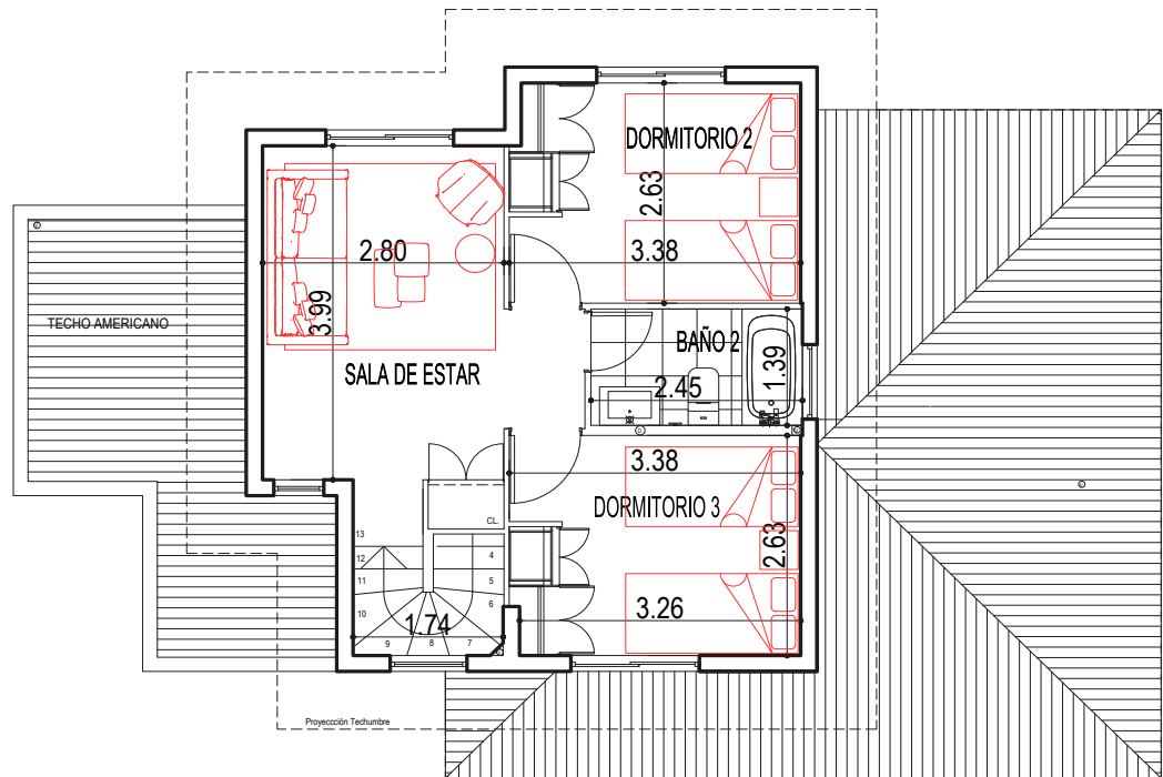
PLANTA SEGUNDO PISO
