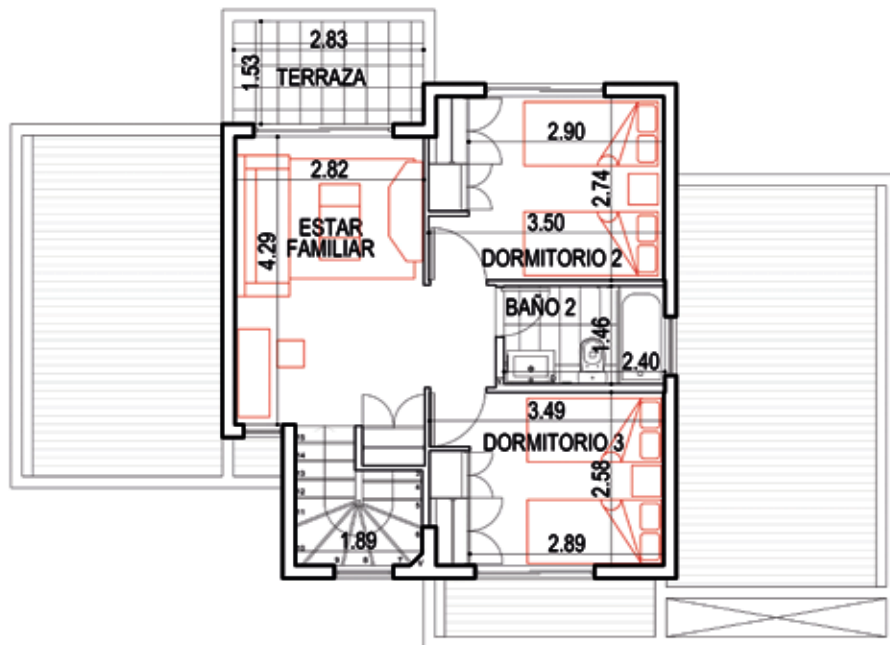
PLANTA SEGUNDO PISO
